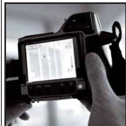
A l'aide d'une caméra spéciale, la thermographie à infrarouges permet d'analyser un bâtiment pour trouver les défauts d'isolation et d'étanchéité. Photos L.Cheviet (à g.) et DER (à dr.).
