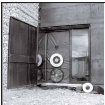
Test d'étanchéité à l'air, à l'aide d'une porte blowerdoor (à g.). En mettant le bâtiment en dépression ou en surpression, on analyse le taux de renouvellement d'air et la perméabilité. Photos DER.
